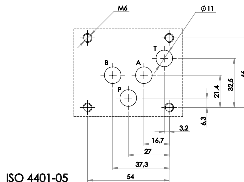
ISO 4401-05
